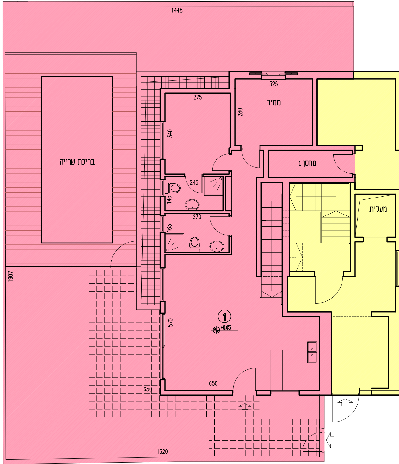
קומה קרקע - תכנית דירה 1 קומה עליונה
